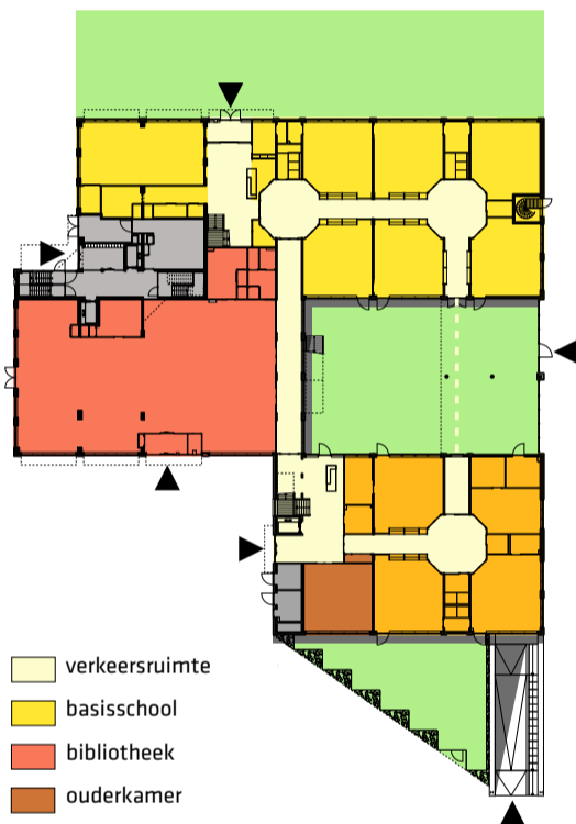
begane grond
