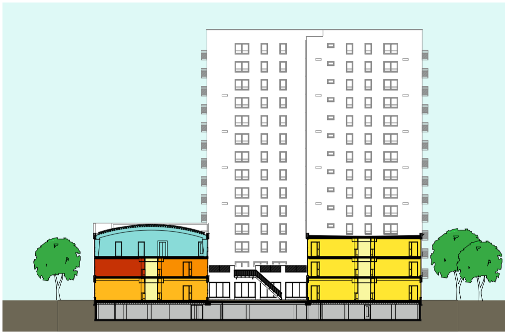
doorsnede
